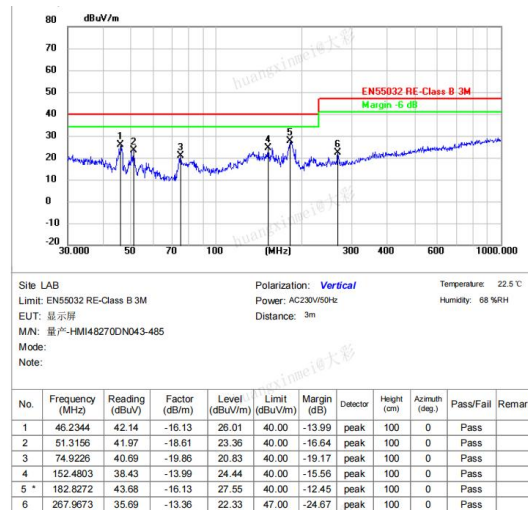
图 4-7 RE 测试垂直方向
