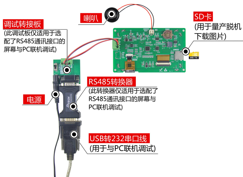
图 1-5 调试工具图
