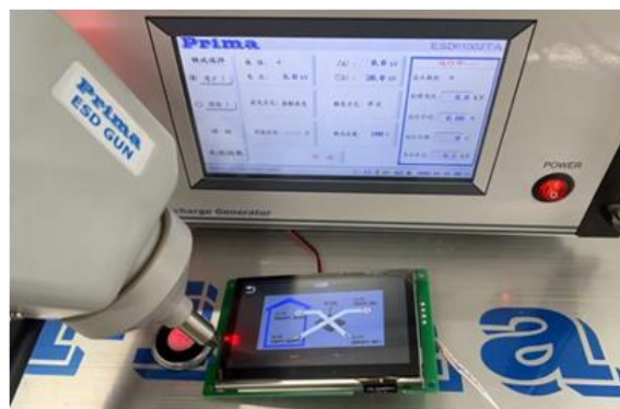
图 4-2 ESD 测试图
