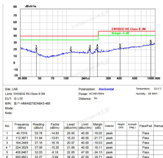
图 4-6 RE 测试水平方向
